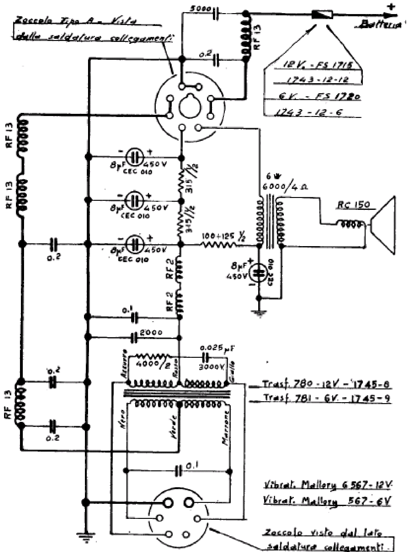
GALLO «CONDOR» - Autoradio mod. SAETTA II - Gruppo alimentatore.
